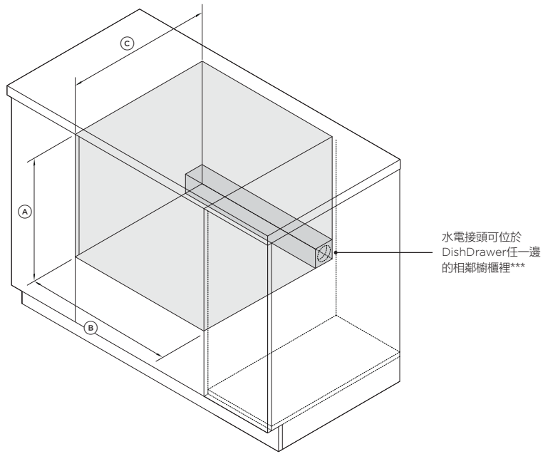
等角視圖
