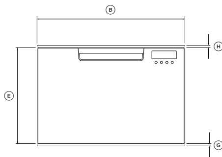
正視圖
