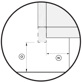
DETAIL 3: SPELING ONDERSTE MEUBELS
